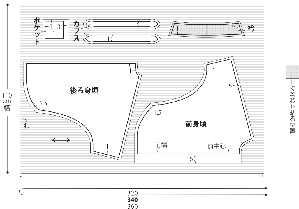
17・18 表布の裁ち方図
